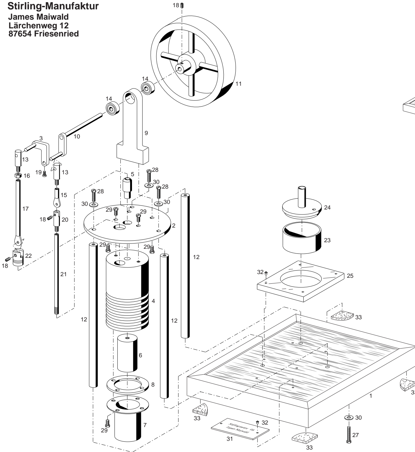
Stückliste/Ersatzteilliste Stirling Motor JM02
